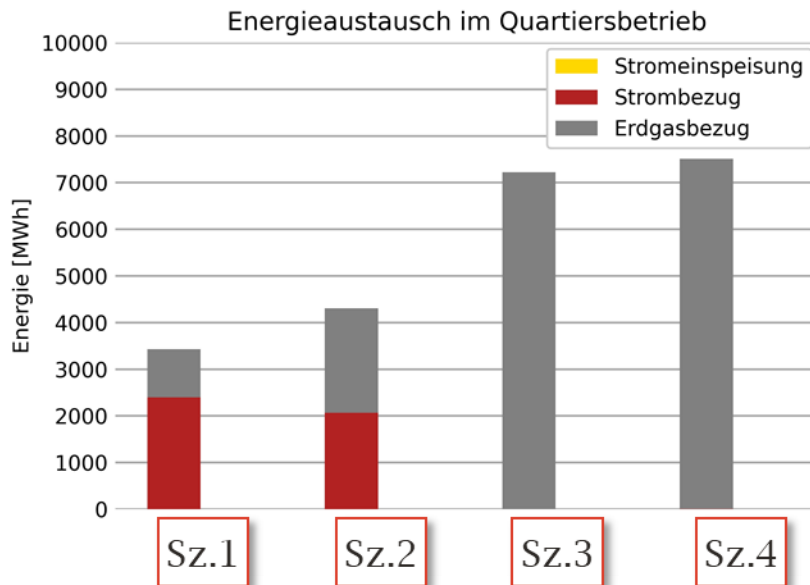
Abbildung 10.13: Energieaustausch im kostenoptimierten Quartiersbetrieb des Städtetzes im sanierten Zustand 2040 mit vollständiger EV-Durchdringung und größeren Pufferspeichern
