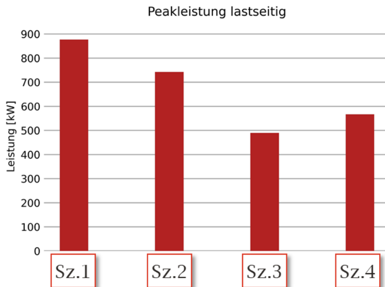
Abbildung 10.2: Lastseitige Peakleistung im kostenoptimierten Quartiersbetrieb des Stadtnetzes mit 50-prozentiger PV-Durchdringung
