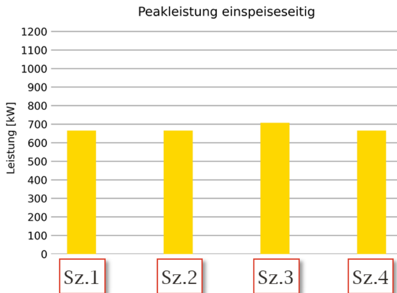
Abbildung 10.20: Einspeiseseitige Peakleistung im systemischen Quartiersbetrieb des Stadtnetzes im sanierten Zustand 2040 mit vollständiger PV-Durchdringung und 50-prozentigem Anteil Batteriespeichern
