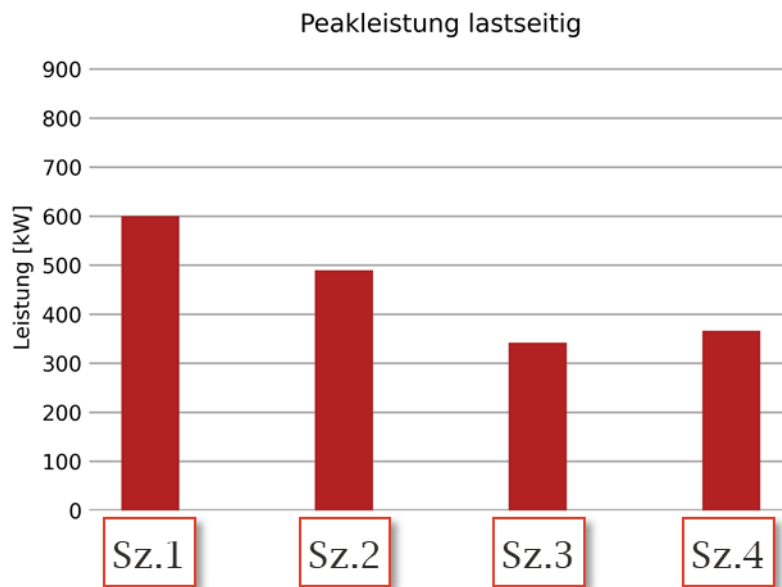
Abbildung 10.4: Peakleistung im systemischen Quartiersbetrieb des Stadtnetzes im sanierten Zustand 2040
