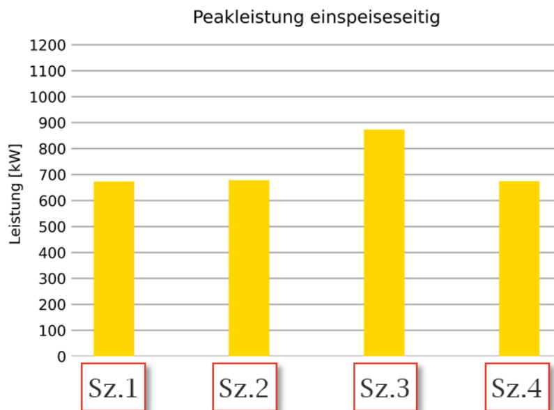
Abbildung 4.13: Einspeiseseitige Peakleistung im kostenoptimierten Quartiersbetrieb des Stadtnetzes mit vollständiger PV-Durchdringung und 50-prozentigem Anteil Batteriespeicher
