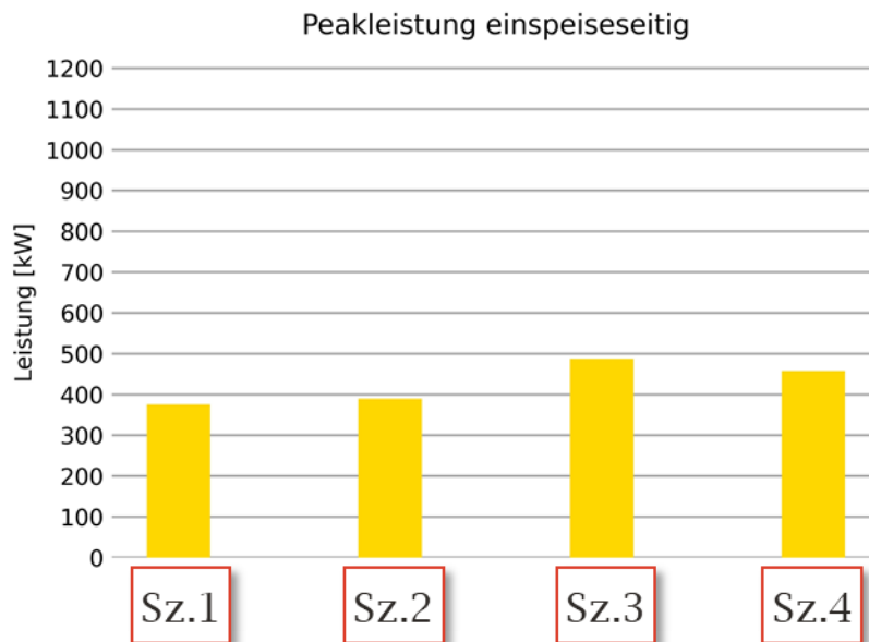
Abbildung 10.14: Einspeiseseitige Peakleistung im kostenoptimierten Quartiersbetrieb des Städtetzes im sanierten Zustand 2040 mit 50-prozentiger PV-Durchdringung
