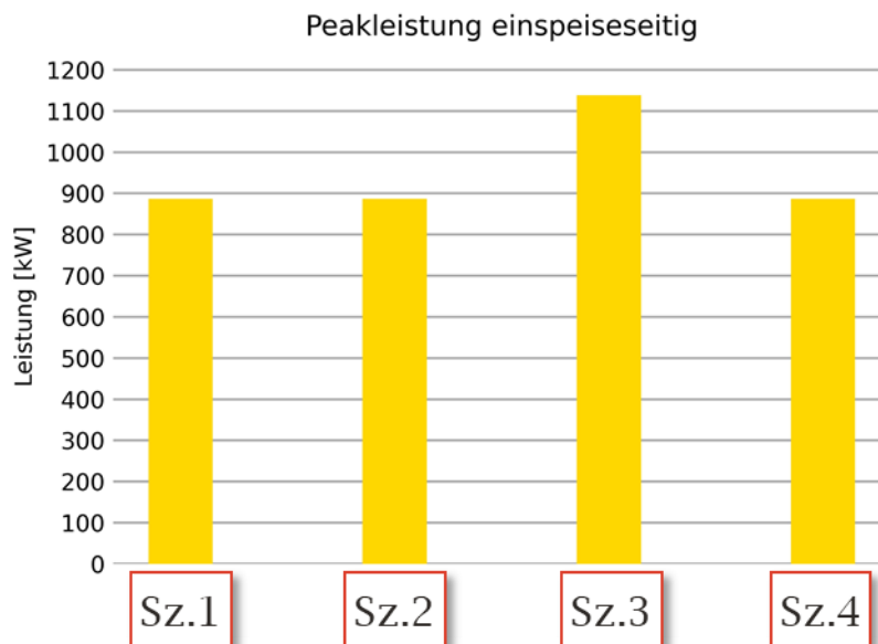
Abbildung 4.15: Einspeiseseitige Peakleistung im kostenoptimierten Quartiersbetrieb des Stadtnetzes mit vollständiger PV-Durchdringung und größeren Pufferspeichern
