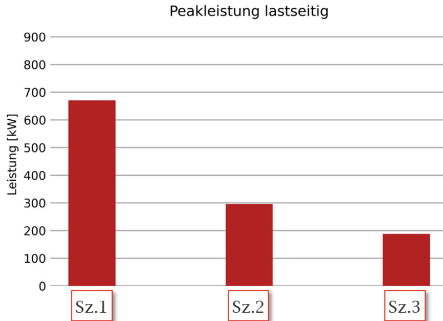
Abbildung 10.29: Peakleistung im kostenoptimierten Quartiersbetrieb des Stadtnetzes im sanierten Zustand 2040 während einer kalten Woche und ohne Berücksichtigung des Haushaltsstrombedarfs
