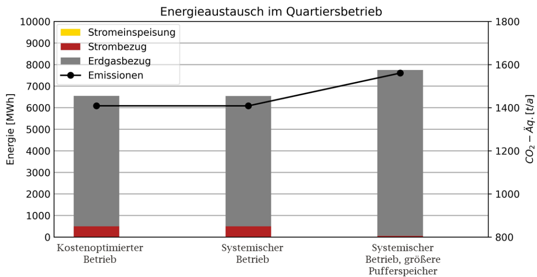
Abbildung 4.6: Energieaustausch und Emissionen in Szenario 4 bei unterschiedlichen Betriebsweisen und thermischen Speicherkapazitäten
