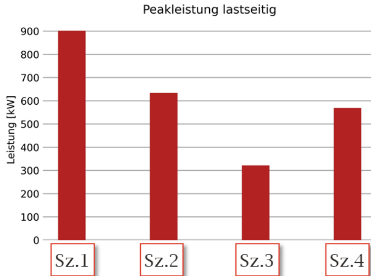
Abbildung 4.1: Peakleistung im kostenoptimierten Quartiersbetrieb des Stadtnetzes
