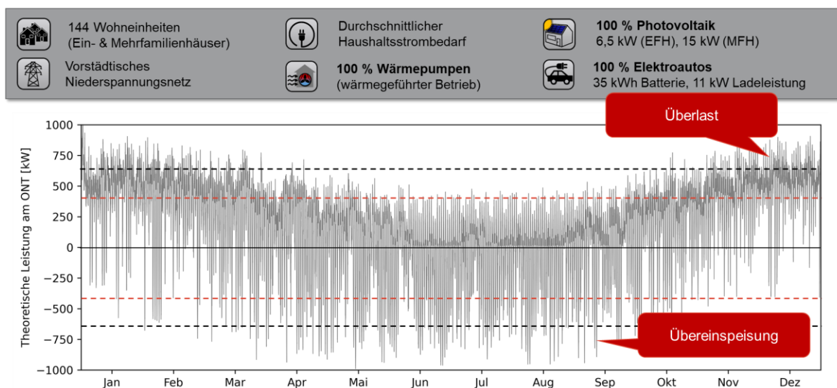
Abbildung 1.1: Auslastung des ONT in einem Vorstadtnetz (rote Linie: extremer ONT, schwarze Linie: typischer ONT) bei einer Technologiedurchdringung von 100 % Wärmepumpen, PV-Anlagen und E-Autos
