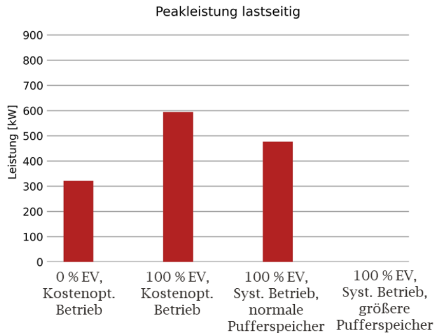
Abbildung 4.7: Peakleistung in Szenario 3 bei unterschiedlichen Betriebsweisen und einer 100-prozentigen E-Auto-Durchdringung
