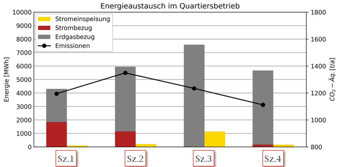
Abbildung 10.3: Energieaustausch und Emissionen im kostenoptimierten Quartiersbetrieb des Stadtnetzes mit 50-prozentiger PV-Durchdringung
